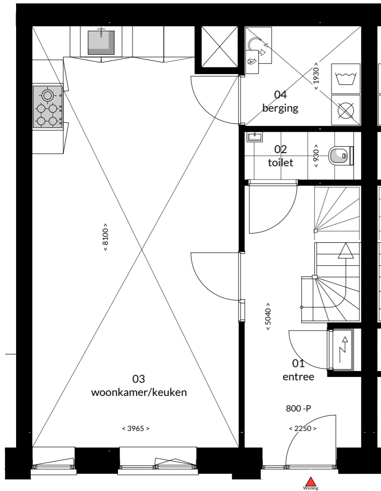
Begane grond
