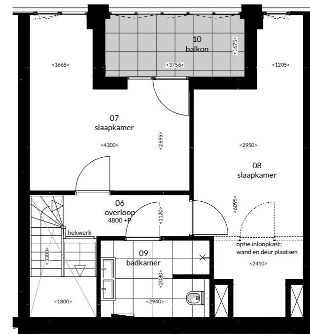
1e verdieping
